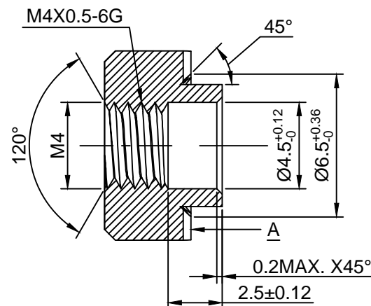
剖面:B-B
